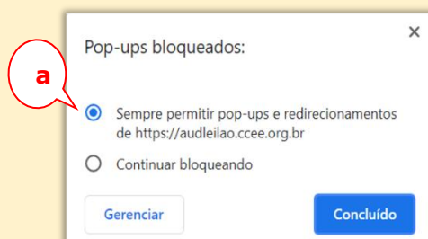
Figura 1 – Desbloquear Pop-ups
